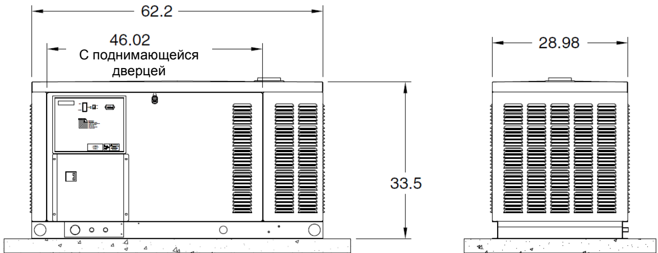
ВИД СПЕРЕДИ
